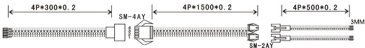
kabel reproduktoru
