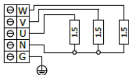
ARI3-45NS-WL 4,5 kW
