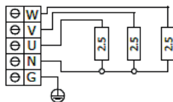
ARI3-75NS-WL 7,5 kW
